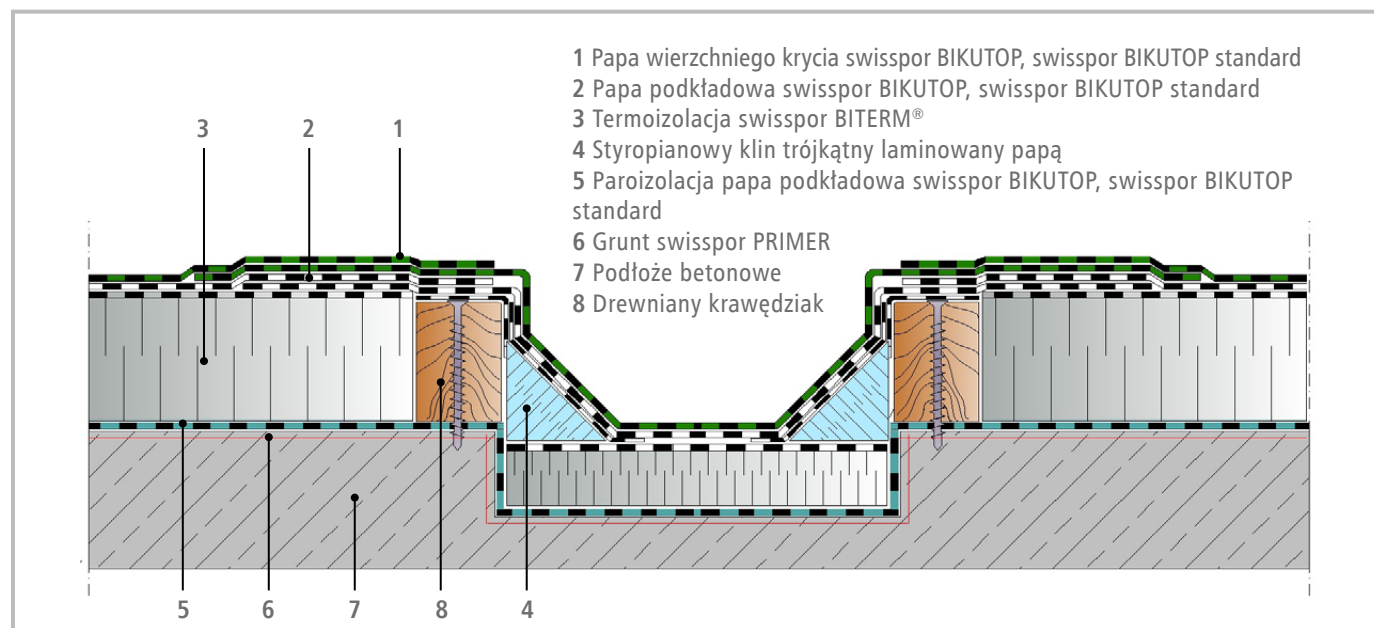
Rys. 51 Obróbka koryta
