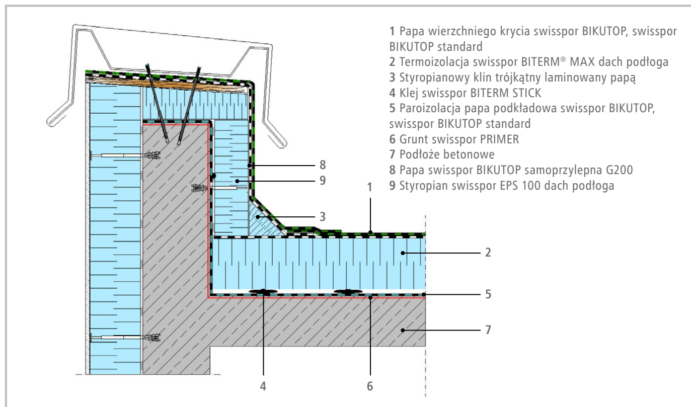
Rys. 45 Obróbka attyki
