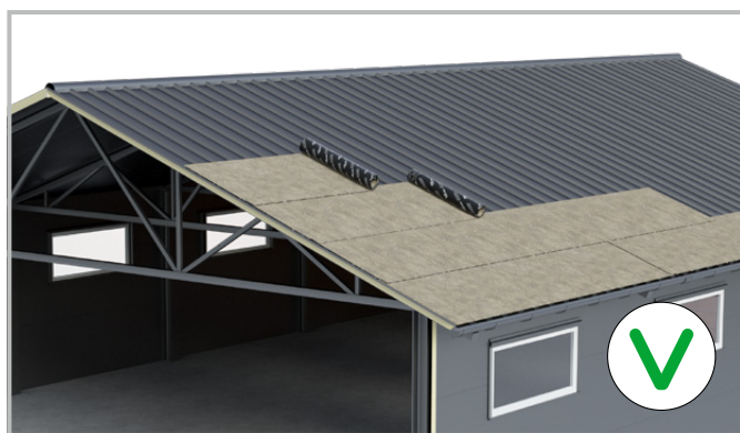
Rys. 3 Kąt nachylenia połaci poniżej 20%
